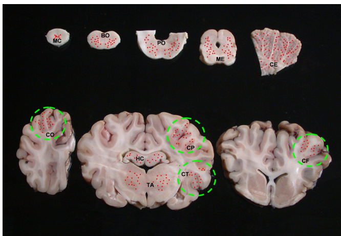
Fig.6. Cortes seriados empregados no estudo histológico e imuno-histoquímico de bovinos com raiva: medula espinal cervical (MC), secção do bulbo na altura do óbex (BO), ponte com pedúnculos cerebelares (PO), mesencéfalo na altura dos colículos rostrais (ME), tálamo (TA), cerebelo (CE), córtex frontal (CF), córtex parietal (CP), córtex temporal (CT), córtex occipital (CO) e hipocampo (HC). Os pontos vermelhos representam os locais de marcação imuno-histoquímica.
